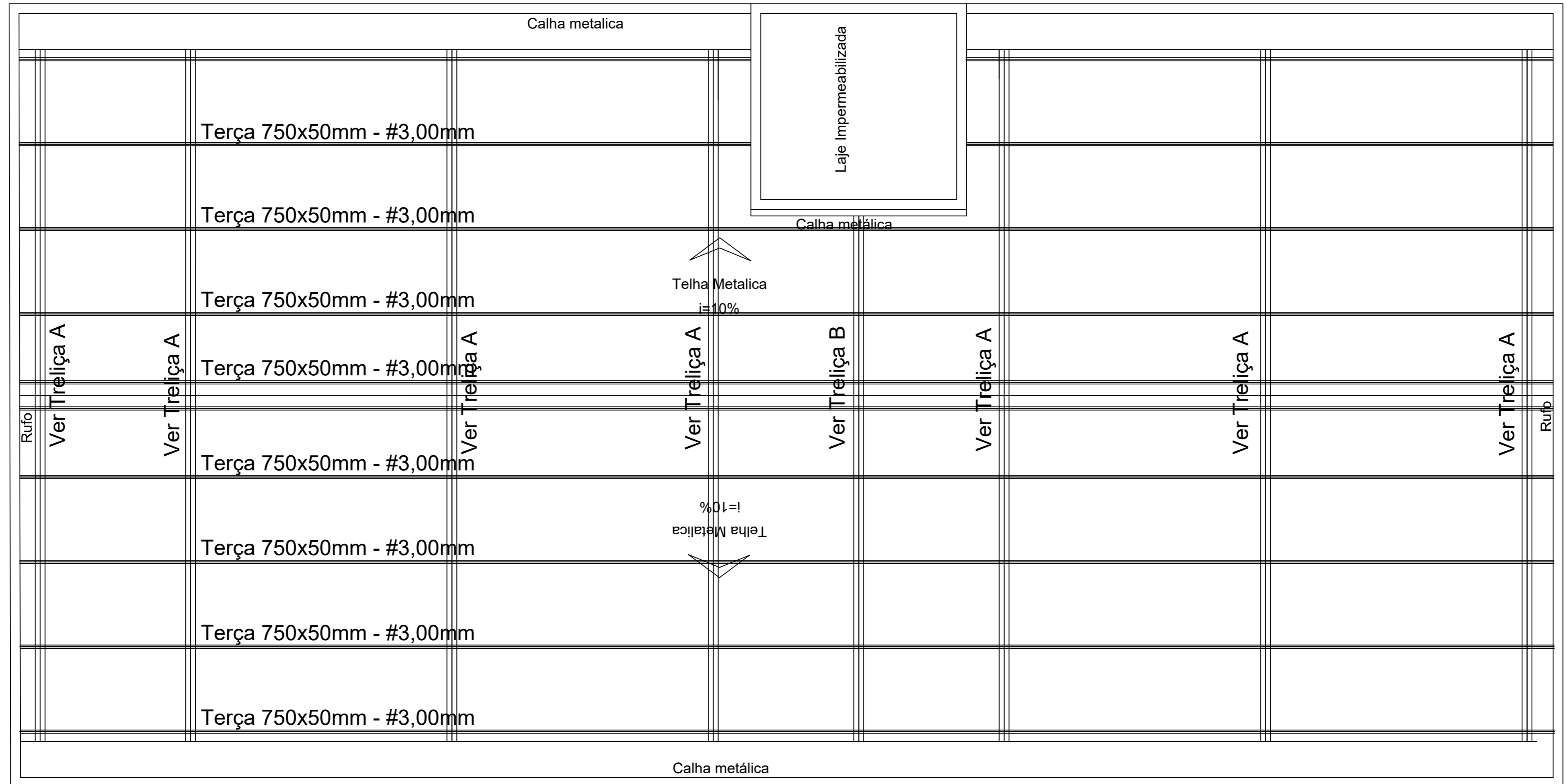
01 PLANTA DE ESTRUTURA METÁLICA Esc. : 1 / 50
